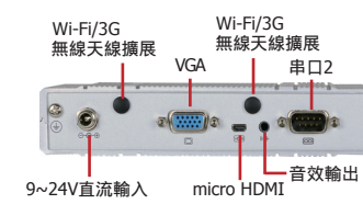
EC800-CD2041-252 後視圖
