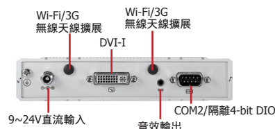
EC800-CD(T)1440-282 EC800-CD1440-252 後視圖
